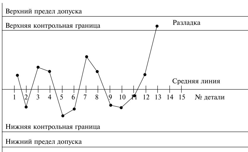
Рис. 10.10. Контрольная карта
